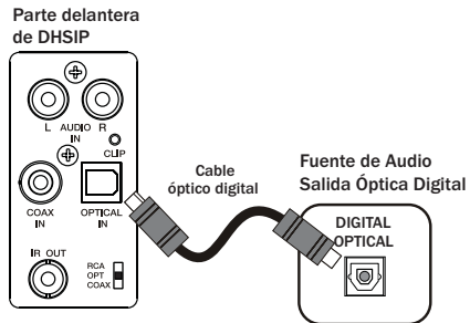
Dibujo 3.2: Fuente de audio a las conexiones ópticas digitales de DHSIP
