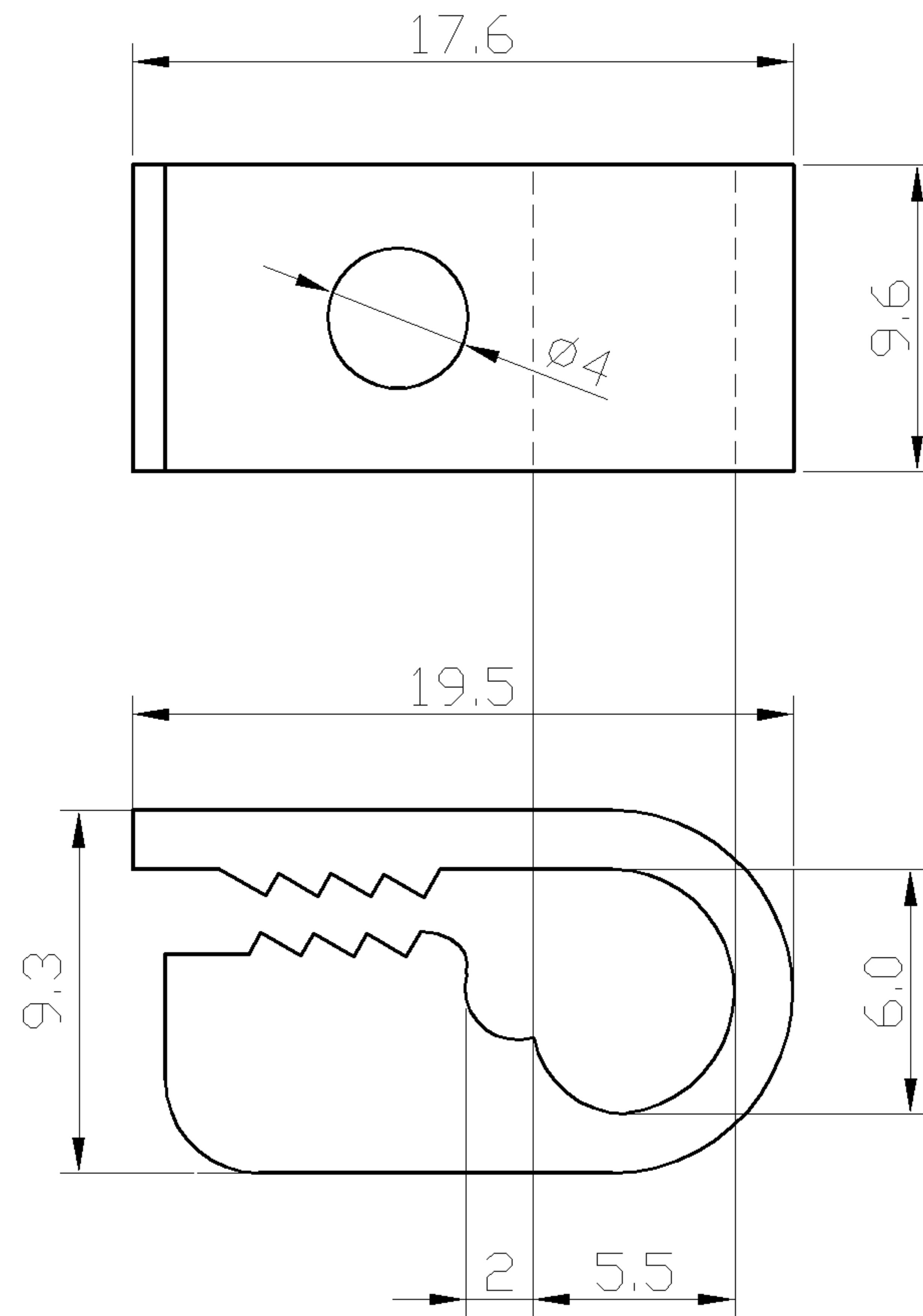
Clip
