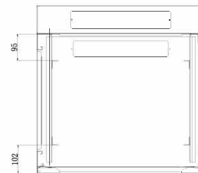
A-A Section
