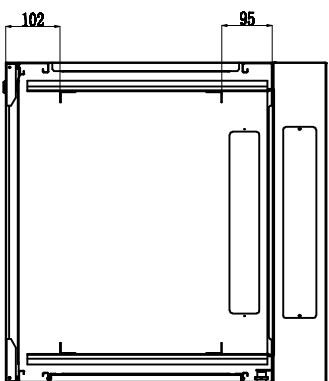
A-A Section
